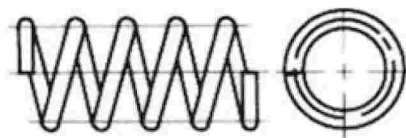
Terminal cerrada sin esmerilar Enrollado izquierdo
